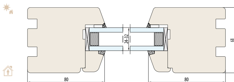
SYSTEM NATURO 68-Fix PRZĘKRÓJ POZIOMY B-B
