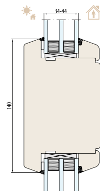
SYSTEM NATURO 80 szpros konstrukcyjny 140 mm
