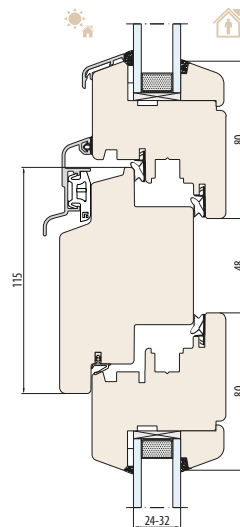
SYSTEM NATURO 68 śleńię 115 mm
