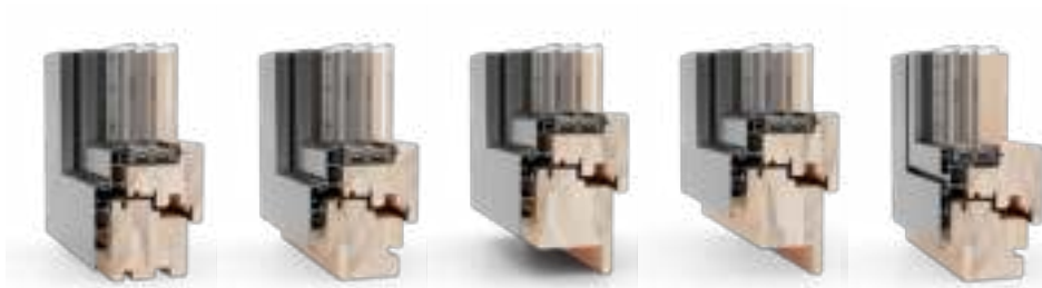
Gemini Classic Profil standardowy (bez podcięcia)
