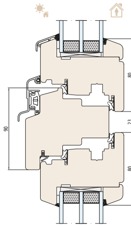
SYSTEM NATURO 92 śleńię 90 mm
