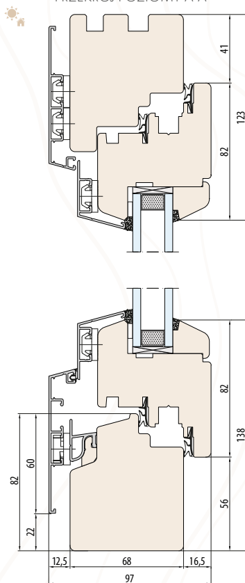
SYSTEM NATURO 68 ALU RENO LINE bez podcięcia pod parapet
