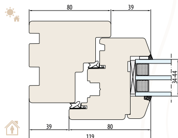
SYSTEM NATURO 80 PRZEKRÓJ POZIOMY B-B
