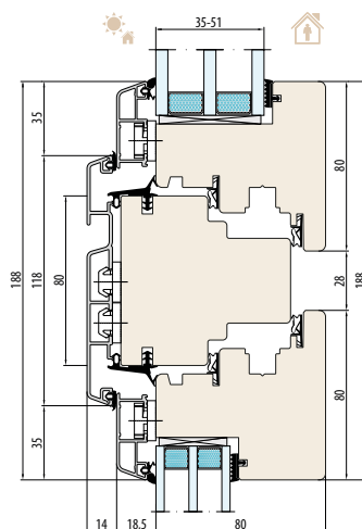
SYSTEM NATURO 80 GEMINI CLASSIC śleńię 80 mm
