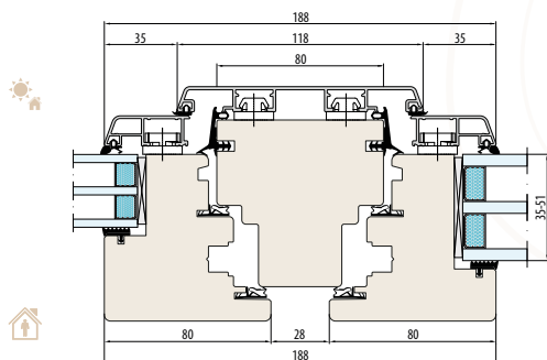
SYSTEM NATURO 80 ALU GEMINI CLASSIC słupki stały 80 mm (przekrój poziomy)
