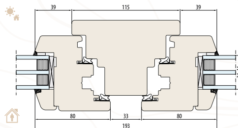
SYSTEM NATURO 80 słupki stały 115 mm (przekrój poziomy)
