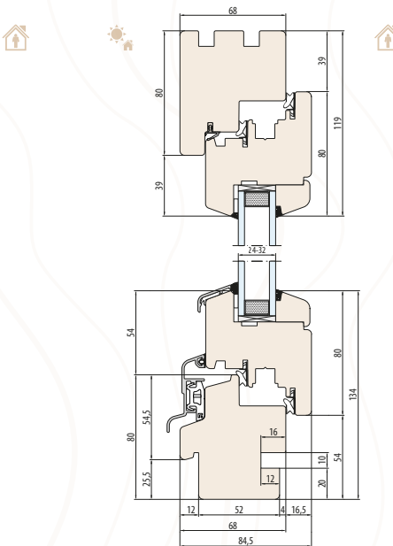
SYSTEM NATURO 68 podcięcie pod parapet wewnętrzne i zewnętrzne
