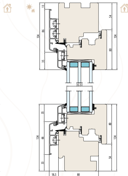
SYSTEM NATURO 80 ALU GEMINI CLASSIC podcięcie pod parapet wewnętrzne i zewnętrzne
