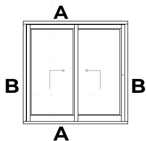
SYSTEM NATURO 68 HST (ogólne wymiary) - próg 22 mm - schemat "D"
