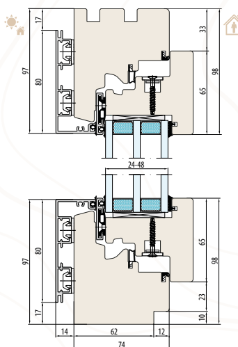
SYSTEM ESPERIA LIFE 74 ALU podcięcie pod parapet wewnętrzne
