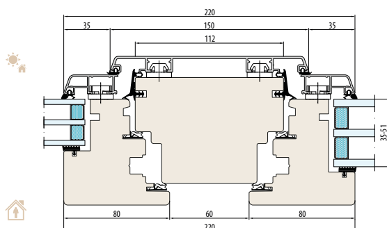
SYSTEM NATURO 80 ALU GEMINI CLASSIC słupki stały 80 mm (przekrój poziomy)
