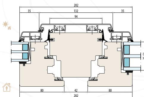
SYSTEM NATURO 80 ALU GEMINI CLASSIC słupki stały 94 mm (przekrój poziomy)
