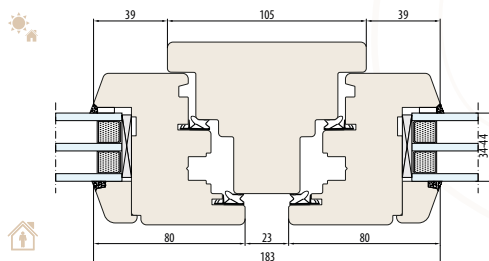
SYSTEM NATURO 80 słupki stały 105 mm (przekrój poziomy)
