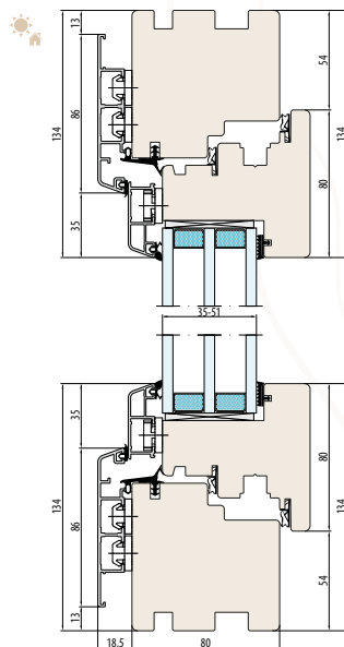
SYSTEM NATURO 80 ALU GEMINI CLASSIC bez podcięcia pod parapet
